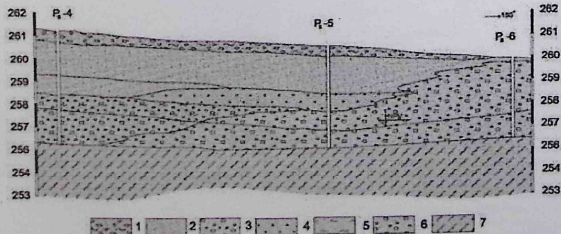
Слика 3. Хидрогеолошки профил терена у подручју изворишта „Лука–Пукли камен“ - Власотинце (по подацима „Геозавада“ - биро Лесковац, 1988.)
