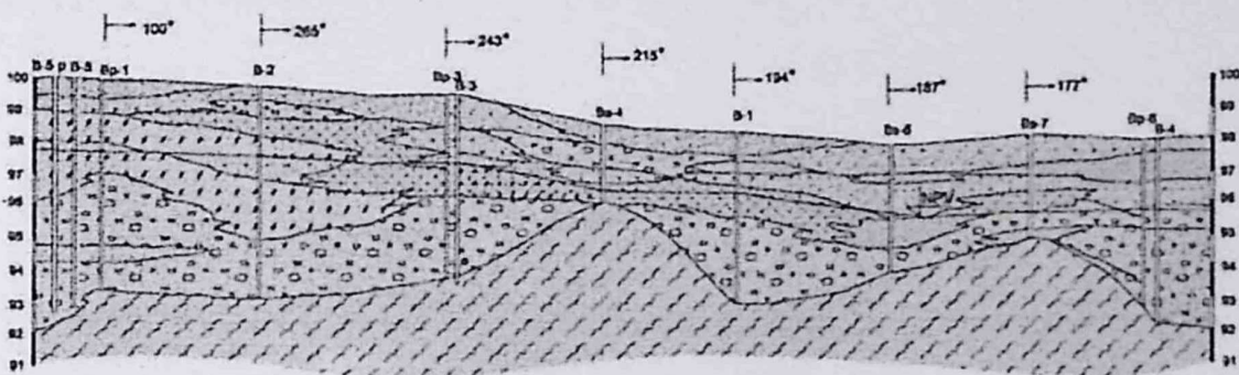
Слика 3. Хидрогеолошки профил терена у подручју изворишта у Бољару
